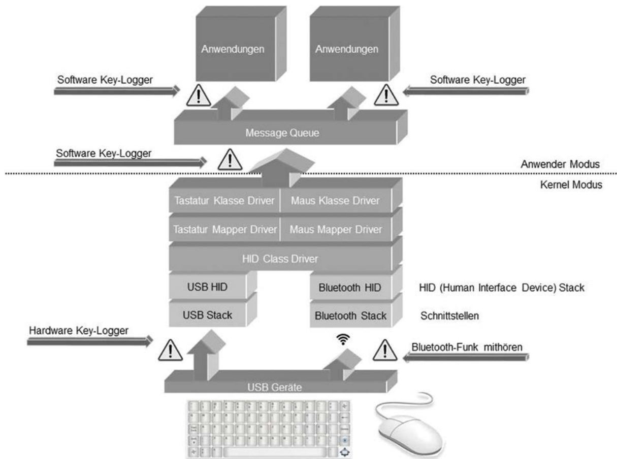
Abbildung 1: Verarbeitung von Eingaben unter Windows (vereinfachte Darstellung)
